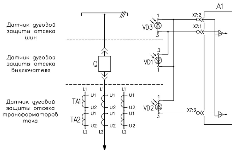
Рисунок 3.1 – Подключение трех датчиков ДДЗ к блоку БЗП-02
