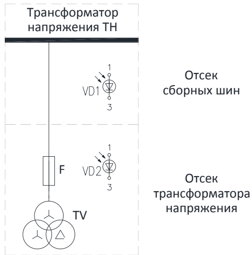
Рисунок 3.2 – Размещение датчиков ДДЗ-01 в ячейке ТН
