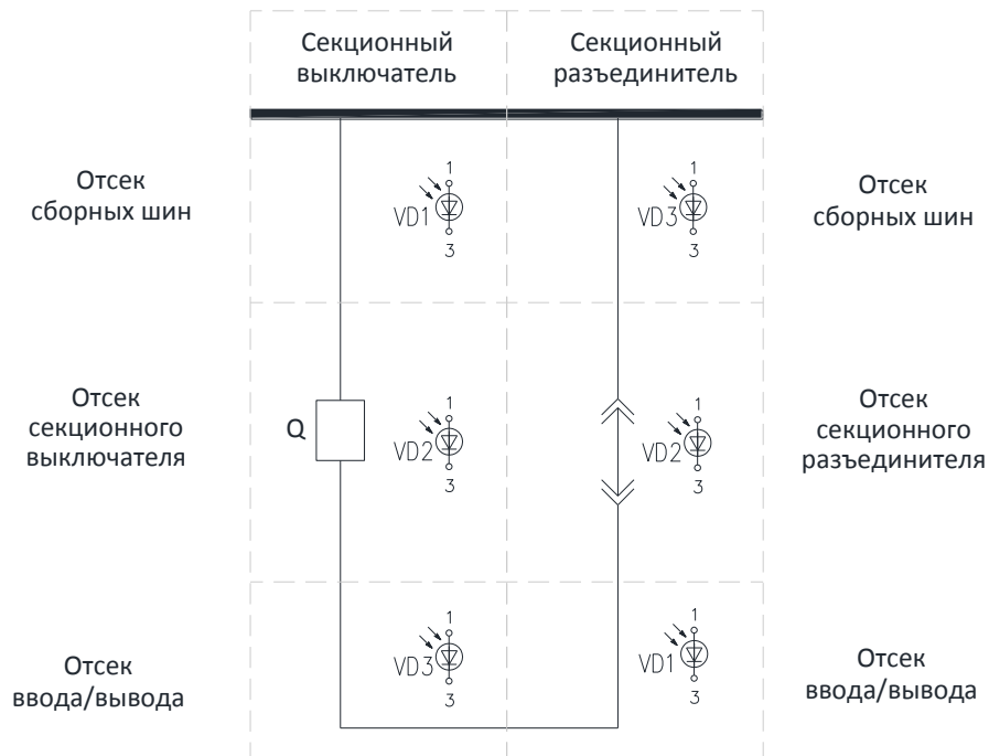
Рисунок 3.3 – Размещение датчиков ДДЗ-01 в ячейке СР
