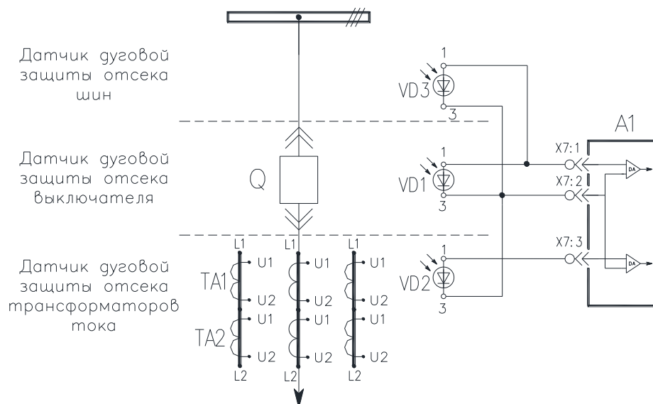
Рисунок 3.1 – Подключение трех датчиков ДДЗ к блоку БЗП-02
