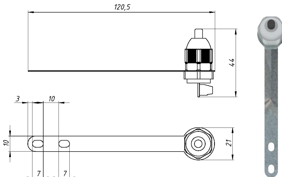
Рисунок 2.1 – Габаритные размеры датчика дуговой защиты
