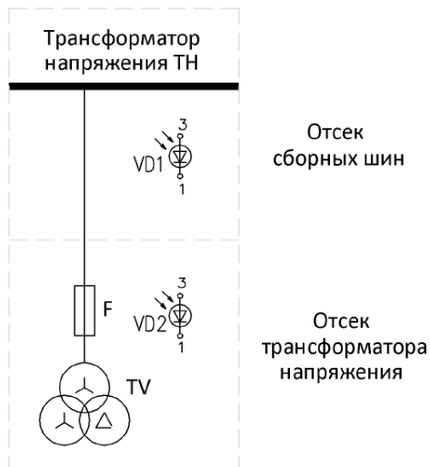
Рисунок 3.2 – Размещение датчиков ДДЗ-01 в ячейке ТН
