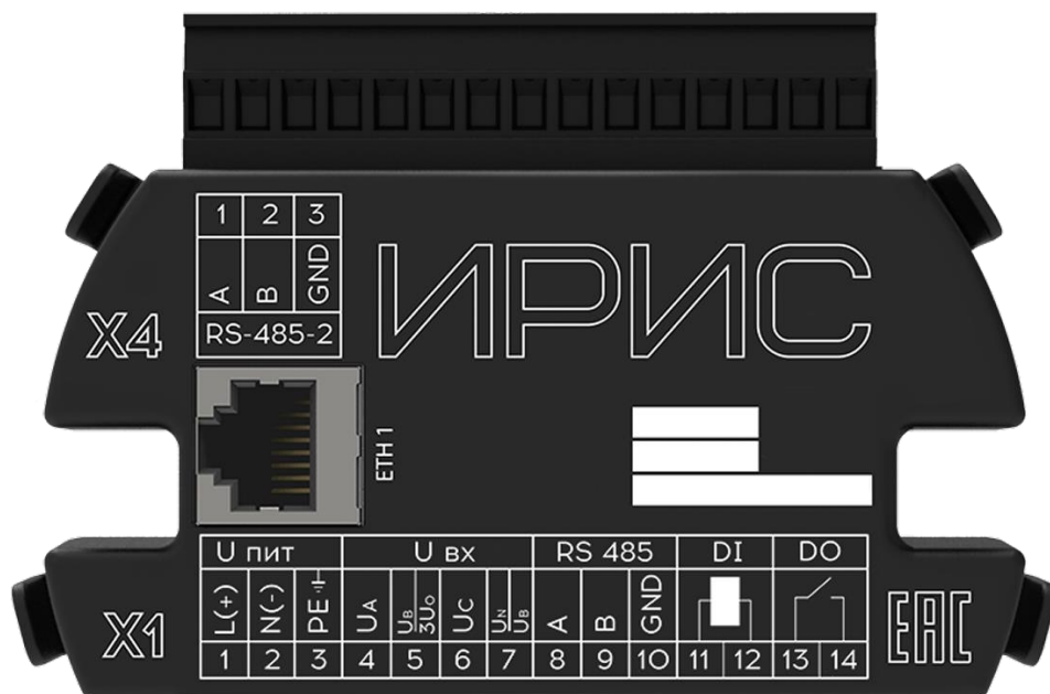
Рисунок 12.10 – Внешний вид рюкзача ИРИС-МИ-ETH
