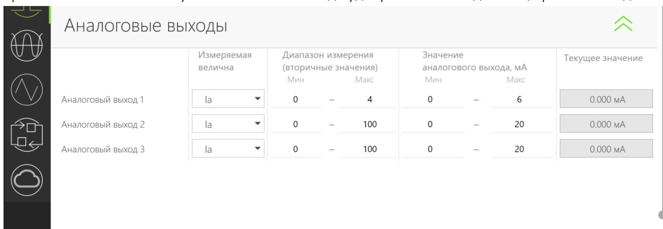
Рисунок 12.4– Пример настройки аналогового выхода
