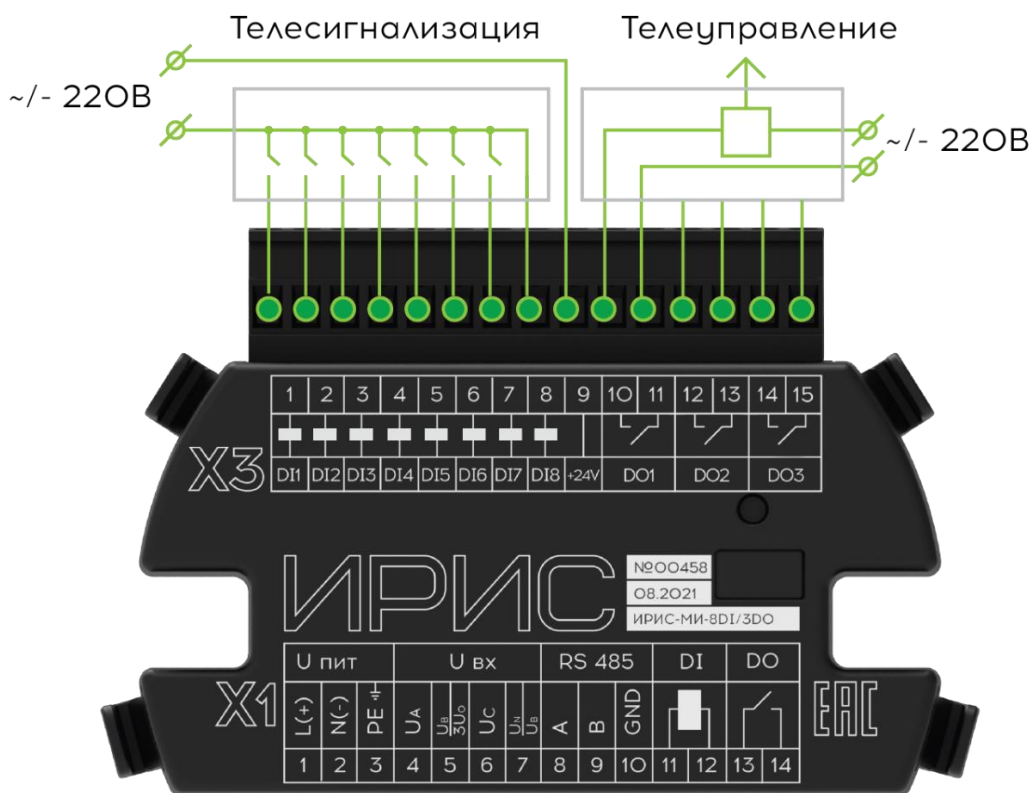
Рисунок 12.8 - Схема подключения рюкзача ИРИС - 8DI/3DO-220V
