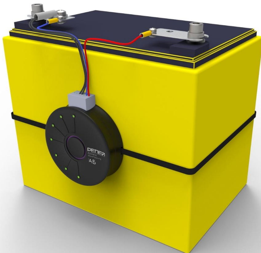
Рисунок В.3. Пример монтажа датчика на один аккумулятор с верхним расположением выводов
