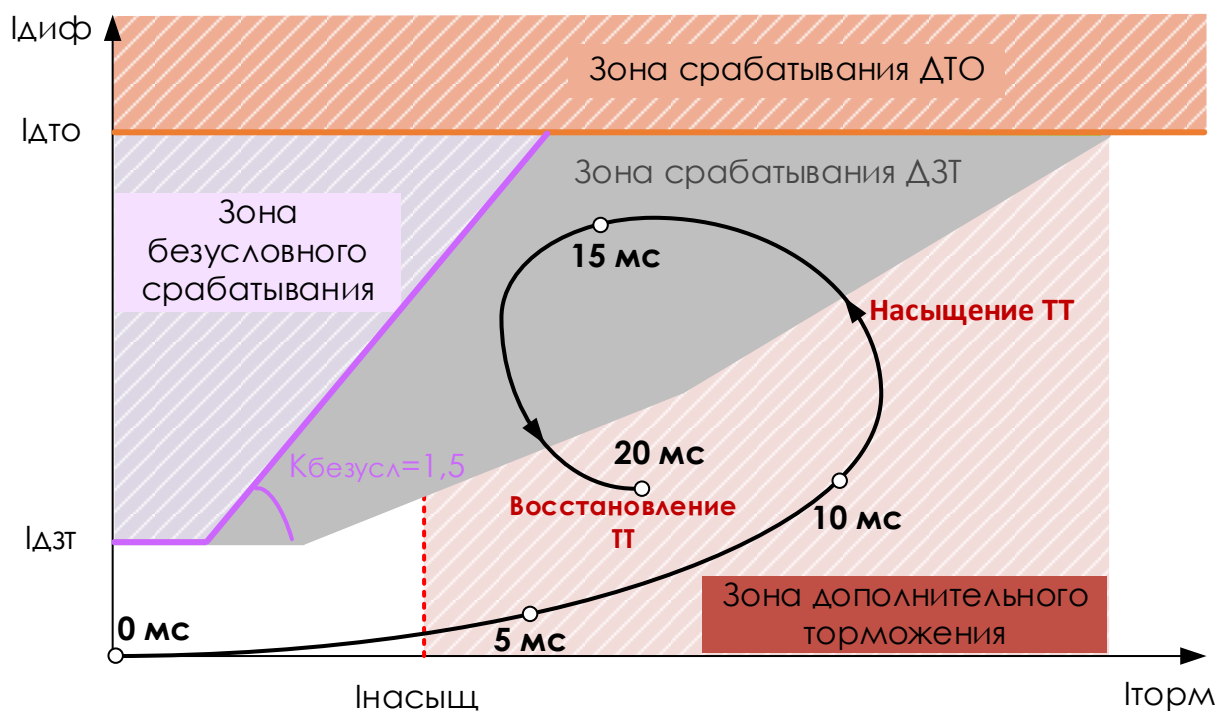
Рисунок 7.3 – Работа ДЗТ при насыщении трансформатора тока
