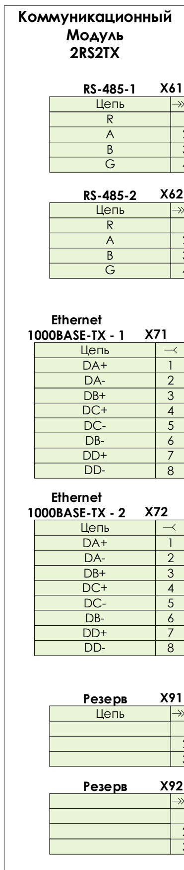
Рисунок 14.3 – Схема электрическая подключения. Часть 2. Коммуникационные модули
