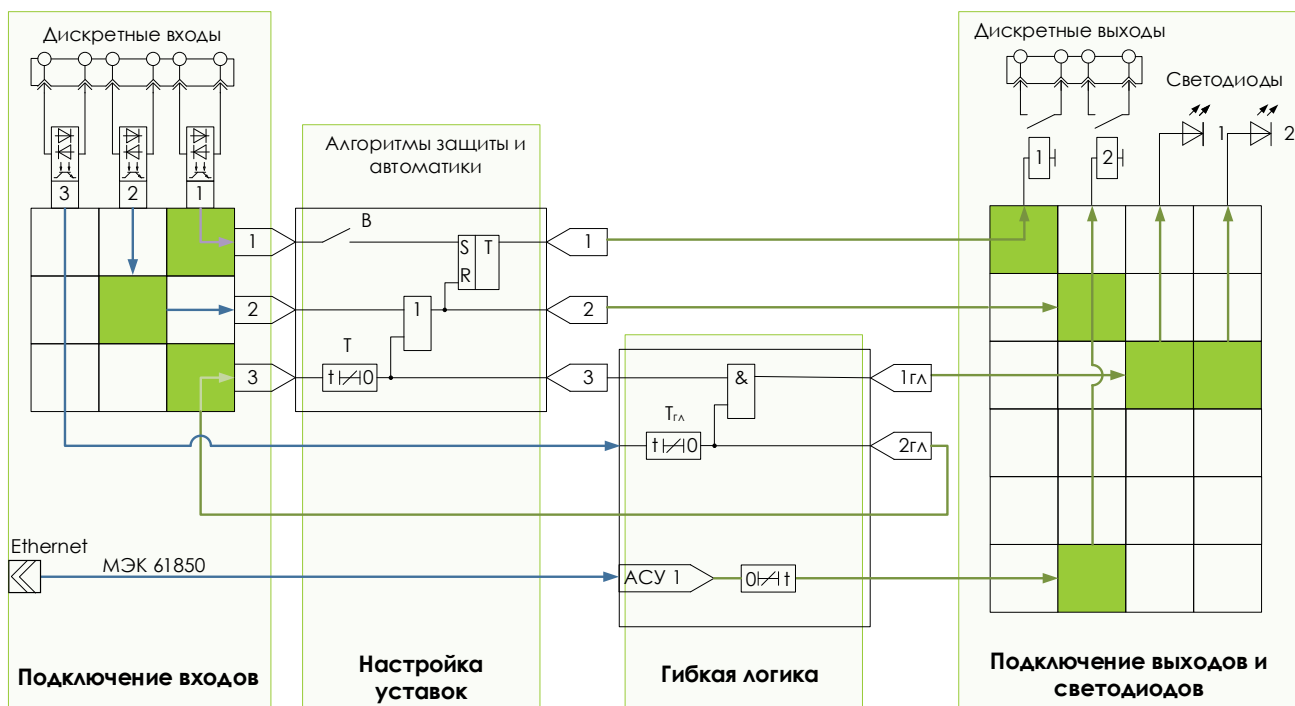
Рисунок 14.1 – Настройка устройства
