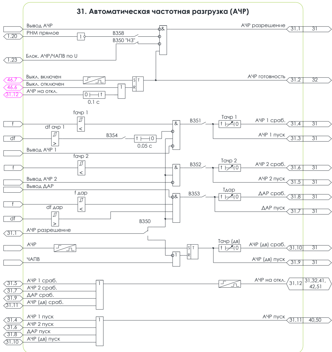
Рисунок 9.1 – Схема №31. Алгоритм АЧР
