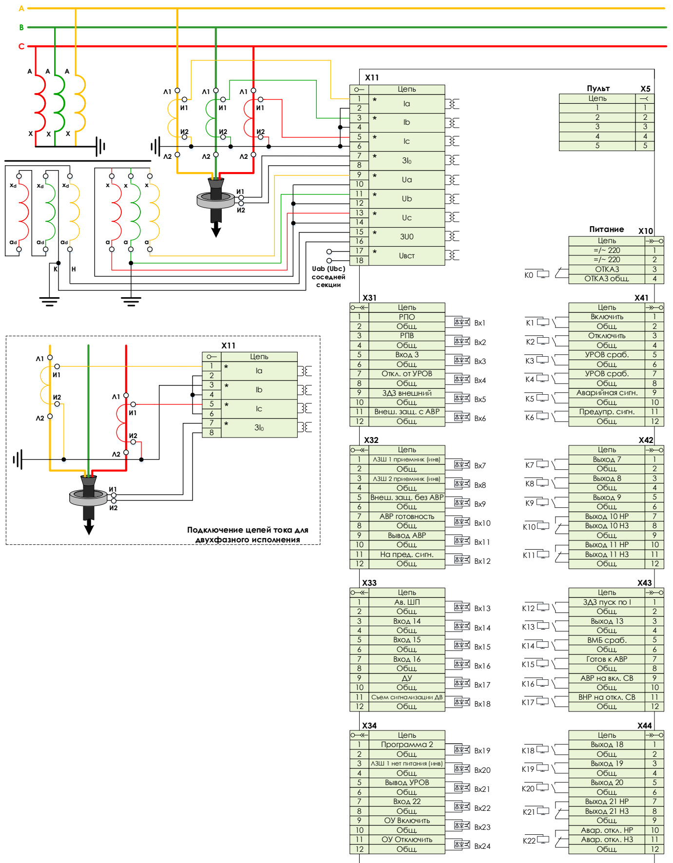
Рисунок 14.5 – Защита на вводном выключателе 6-10 кВ
