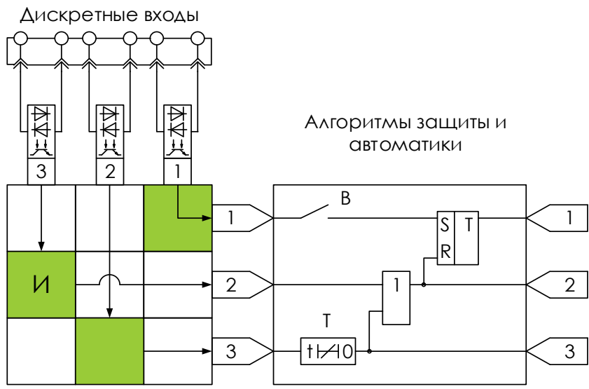
Рисунок 5.1 – Подключение дискретных входов
