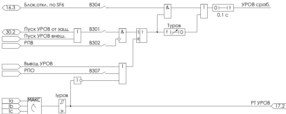
Рисунок 4.22 – Алгоритм УРОВ
