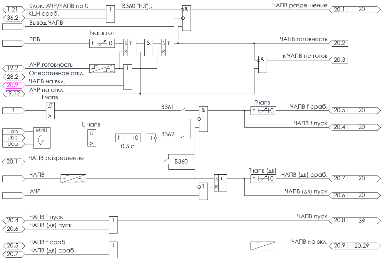
Рисунок 4.24 – Алгоритм ЧАПВ
