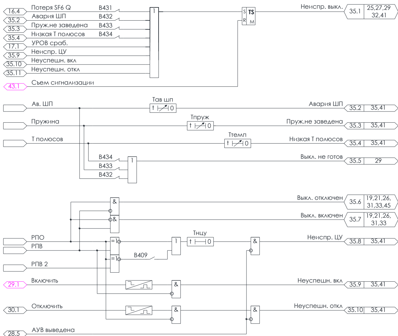
Рисунок 4.38 – Алгоритм диагностики выключателя
