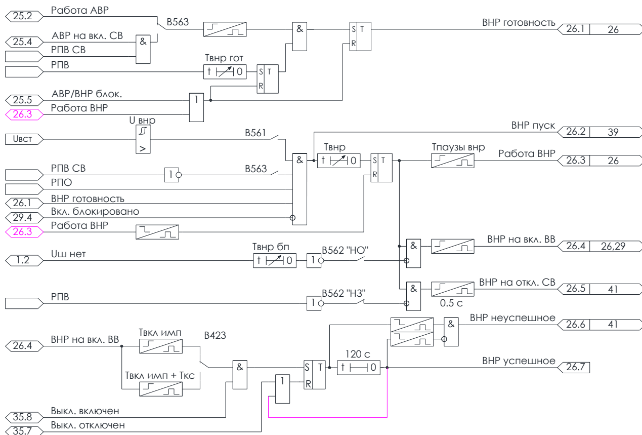
Рисунок 4.30 – Алгоритм ВНР
