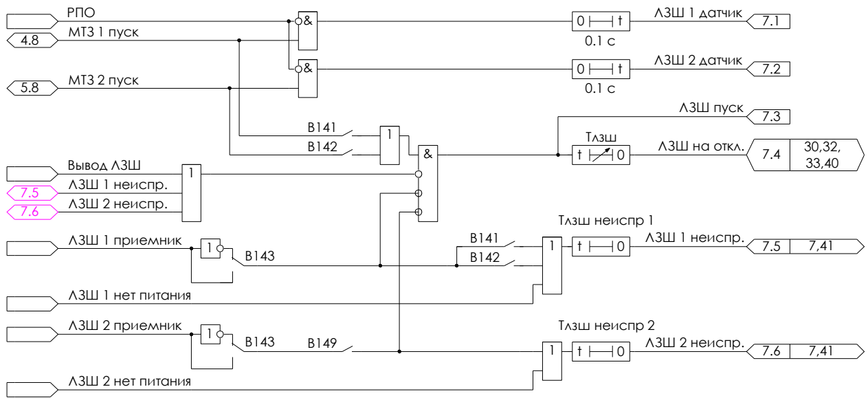
Рисунок 4.11 – Алгоритм ЛЗШ
