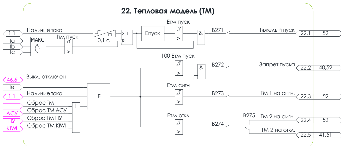
Рисунок 7.2 – Схема №22. Алгоритм ТМ
