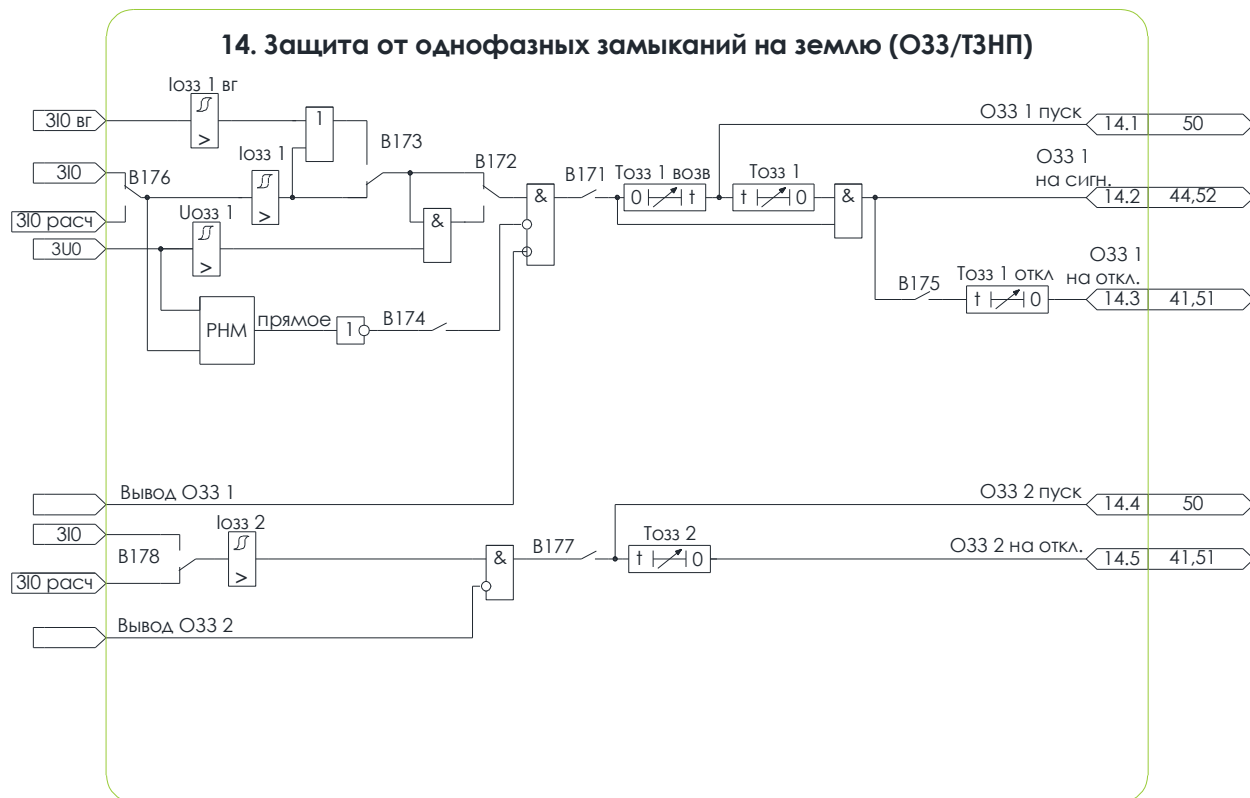
Рисунок 5.9 – Схема №14. Алгоритм ОЗЗ/ТЗНП
