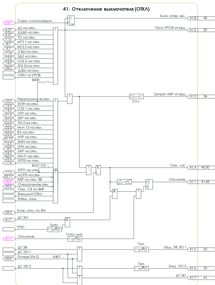
Рисунок 11.3 – Схема №41. Алгоритм отключения выключателя
