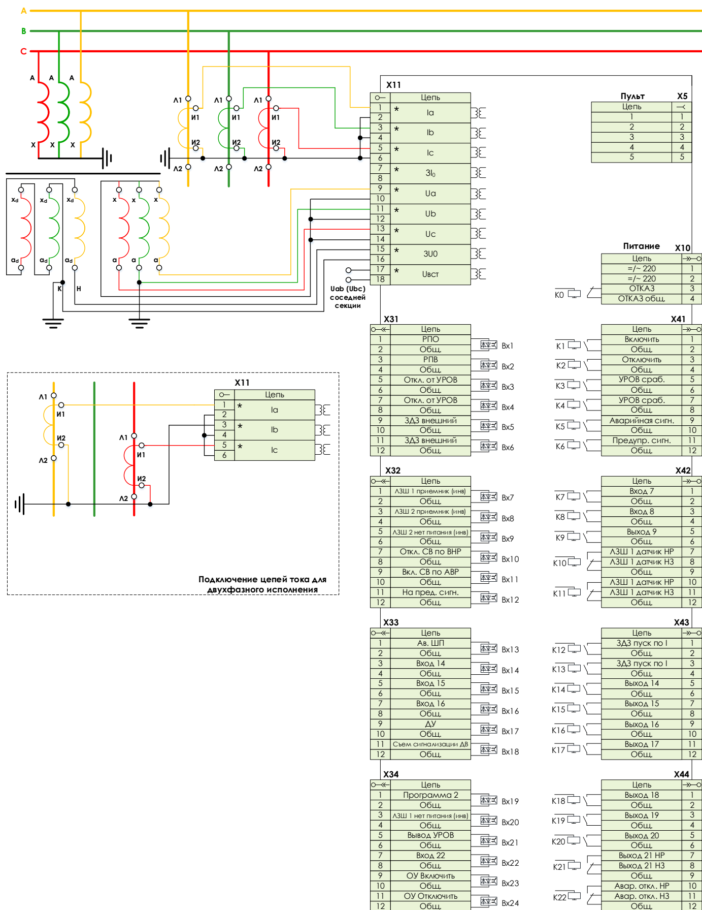
Рисунок 14.6 – Защита на секционном выключателе 6-10 кВ
