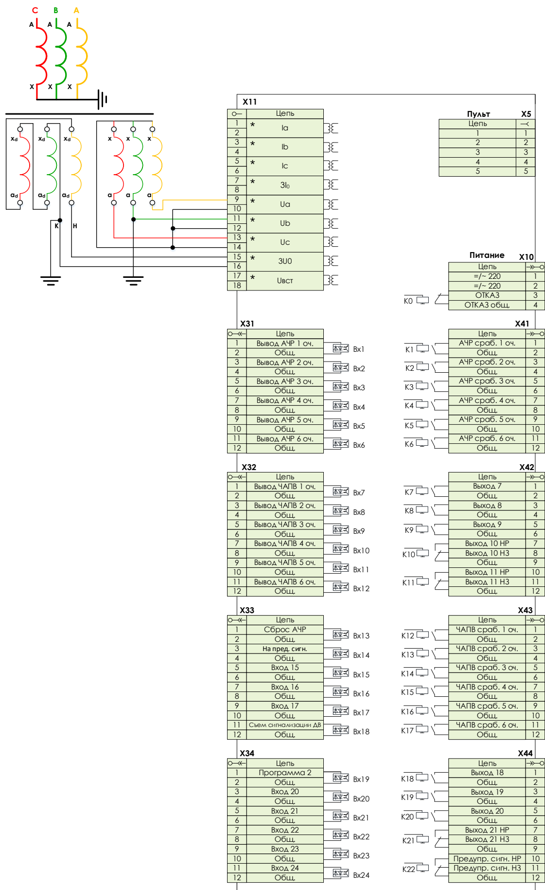
Рисунок 14.8 – Централизованная частотная автоматика
