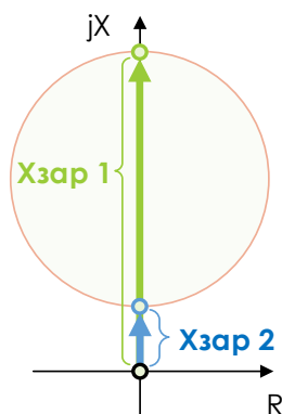
Рисунок 7.5 – Характеристик срабатывания РС ЗАР
