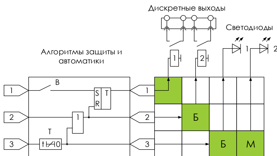
Рисунок 14.11 – Подключение дискретных выходов и светодиодов
