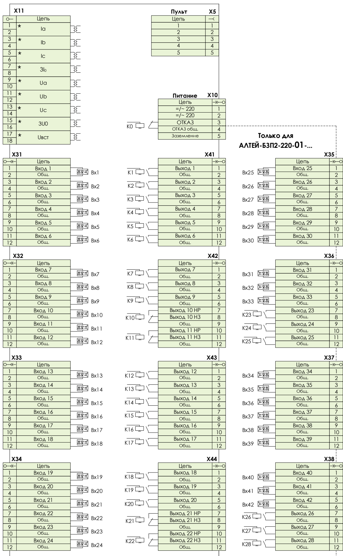
Рисунок 14.2 – Схема электрическая подключения. Часть 1
