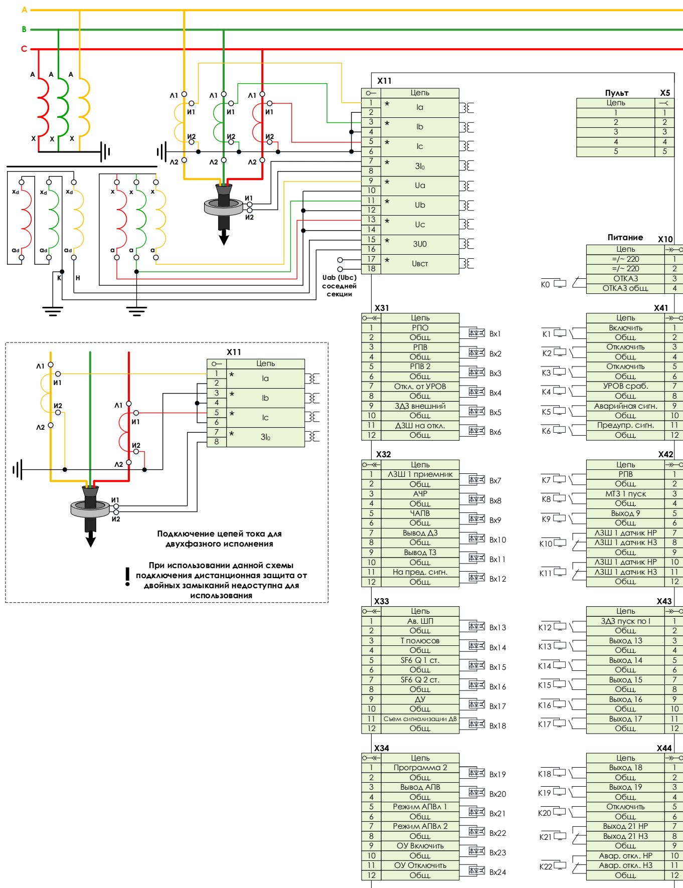
Рисунок 14.9 – Дистанционная защита линии 35 кВ
