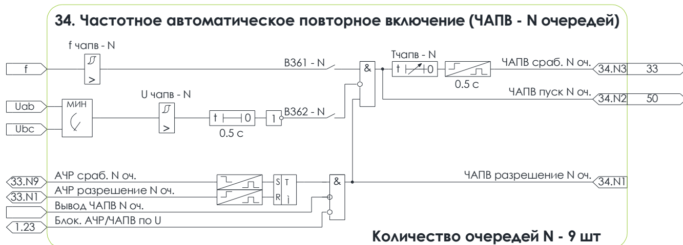
Рисунок 9.4 – Схема №34. Алгоритм ЧАПВ
