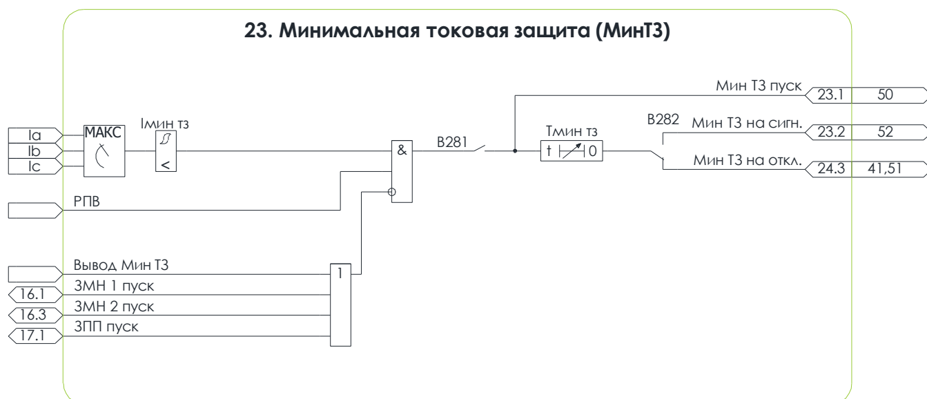
Рисунок 7.3 – Схема №23. Алгоритм МинТЗ
