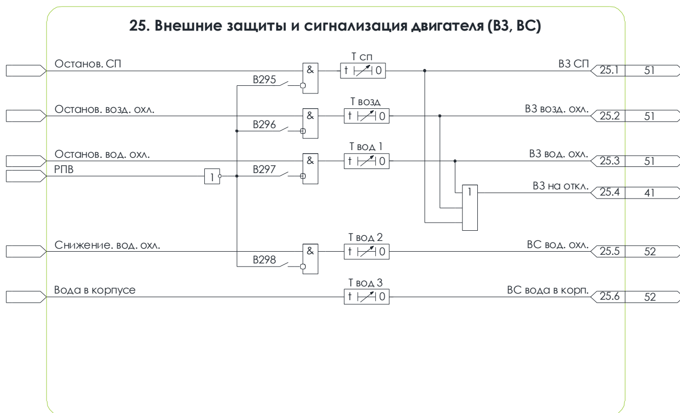
Рисунок 7.6 – Схема №25. Алгоритм ВЗ, ВС
