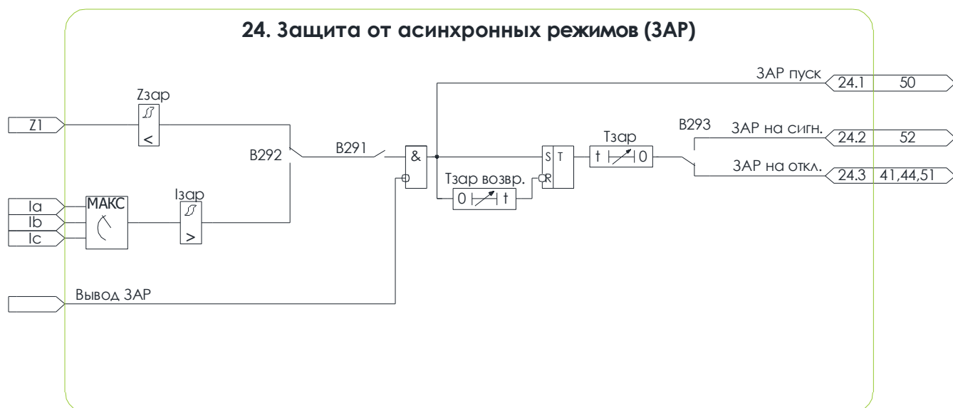
Рисунок 7.4 – Схема №24. Алгоритм ЗАР
