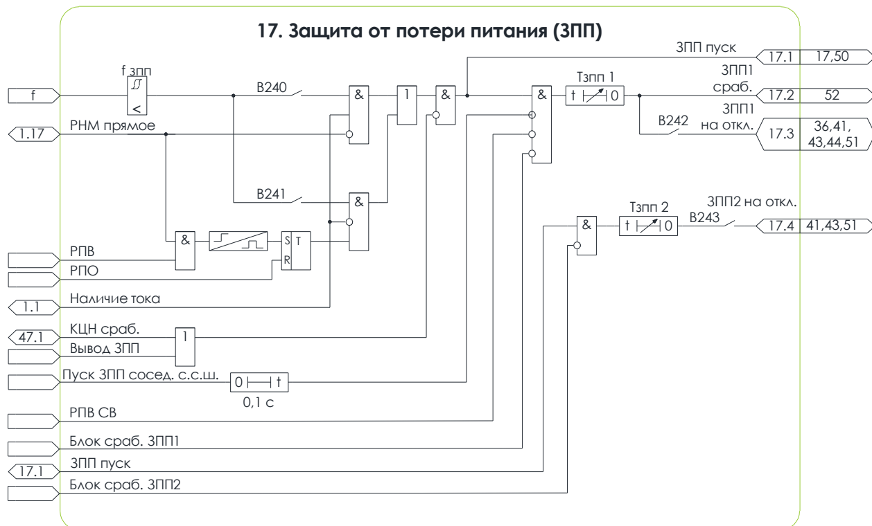
Рисунок 6.2 – Схема №17. Алгоритм ЗПП
