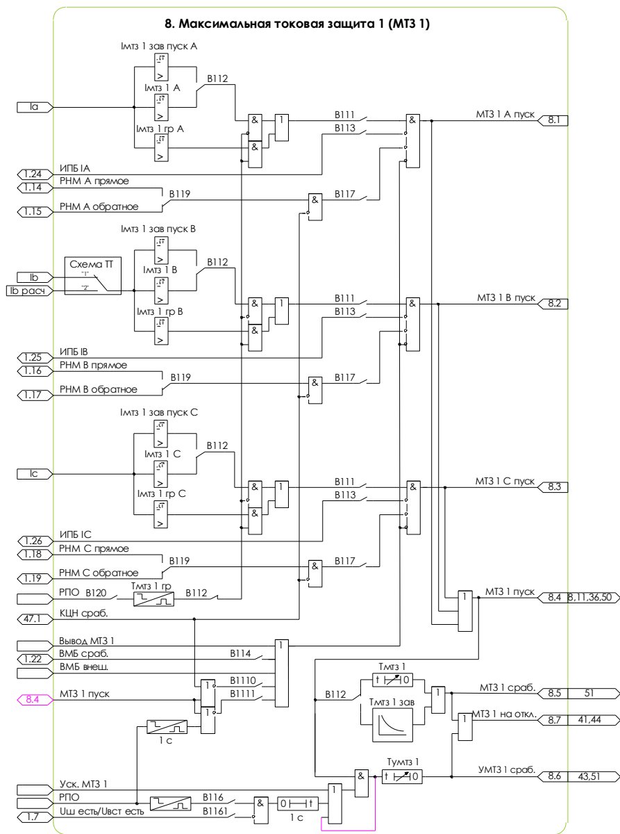
Рисунок 5.2 – Схема №8. Алгоритм МТЗ 1
