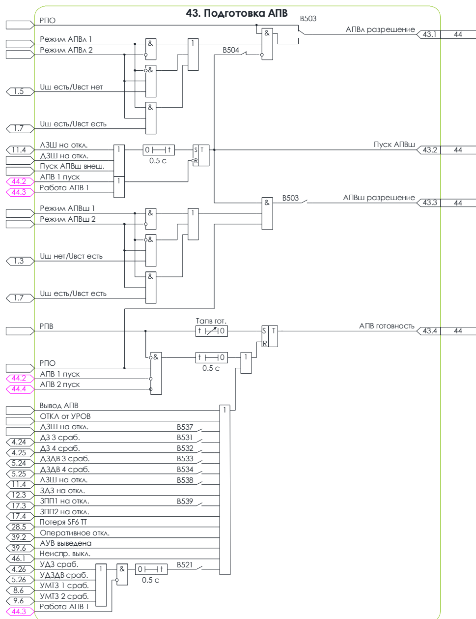
Рисунок 11.5 – Схема №43. Алгоритм подготовки АПВ
