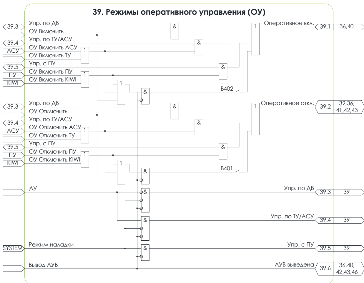
Рисунок 11.1 – Схема №39. Алгоритм ОУ
