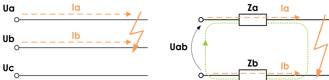
Рисунок 13.3 – Принципиальная схема при двухфазном КЗ
