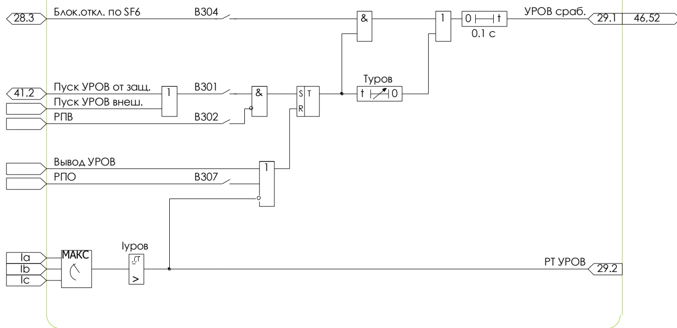
Рисунок 8.2 – Схема №29. Алгоритм УРОВ
