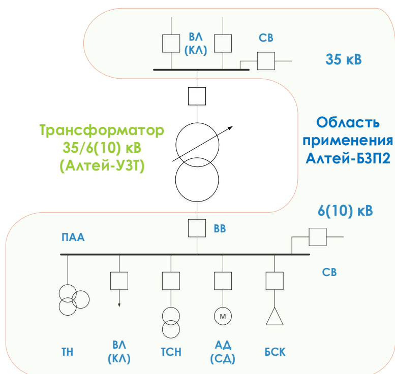
Рисунок 1.1 – Область применения Алтей-БЗП2
