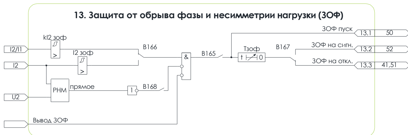
Рисунок 5.8 – Схема №13. Алгоритм ЗОФ
