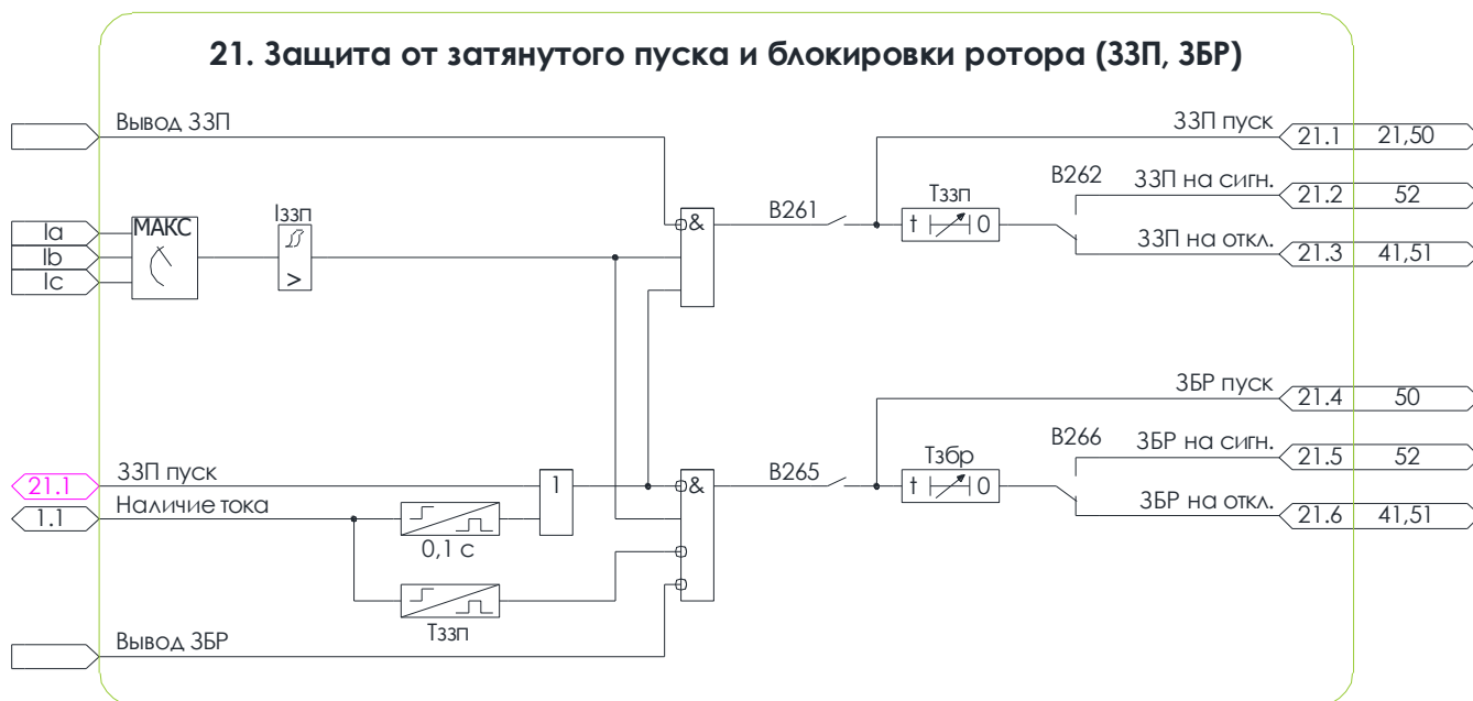
Рисунок 7.1 – Схема №21. Алгоритм 3ЗП, 3БР
