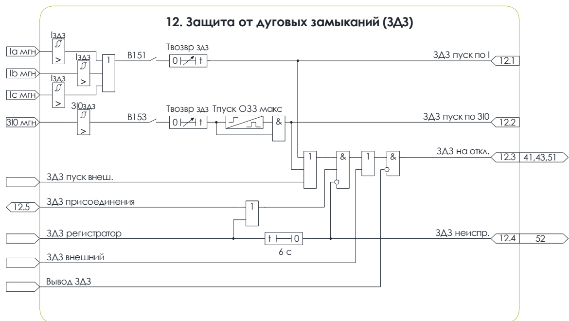
Рисунок 5.7 – Схема №12. Алгоритм ЗДЗ
