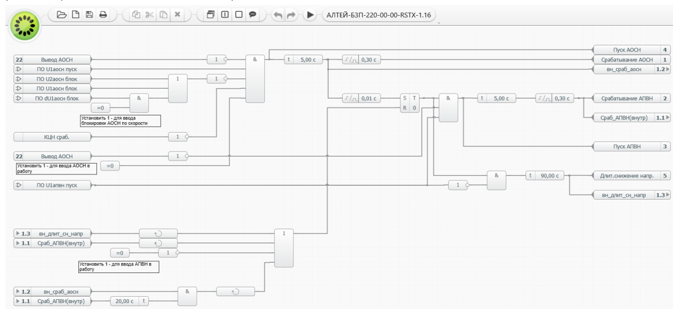
Рисунок 13.7 – Алгоритм АОСН и АПВН в редакторе гибкой логики
