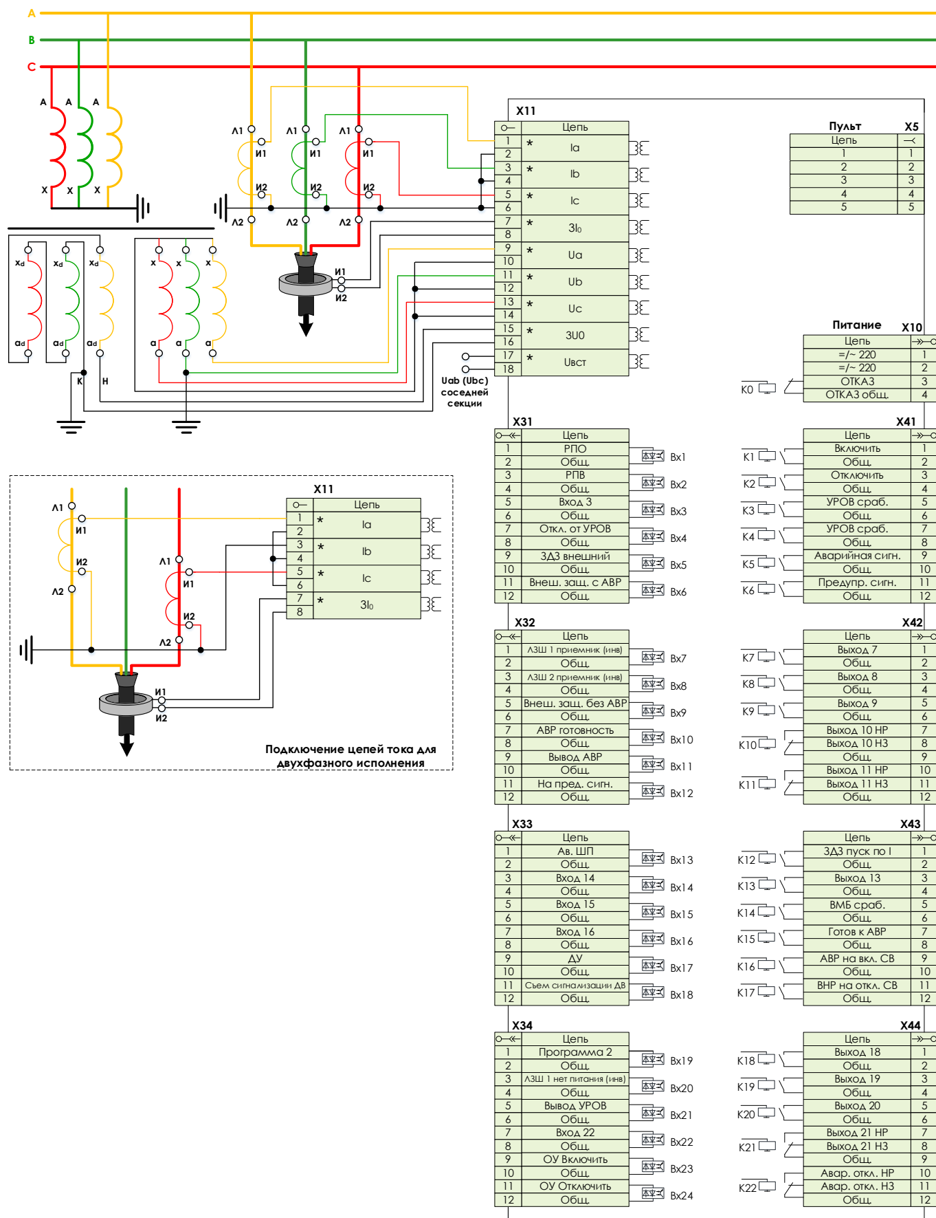
Рисунок 14.5 – Защита на вводном выключателе 6-10 кВ
