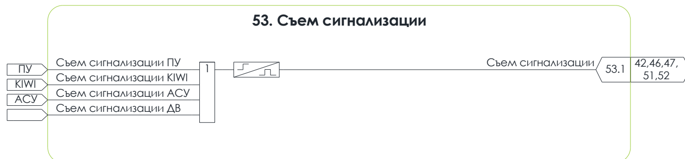
Рисунок 13.6 – Схема №53. Алгоритм съема сигнализации
