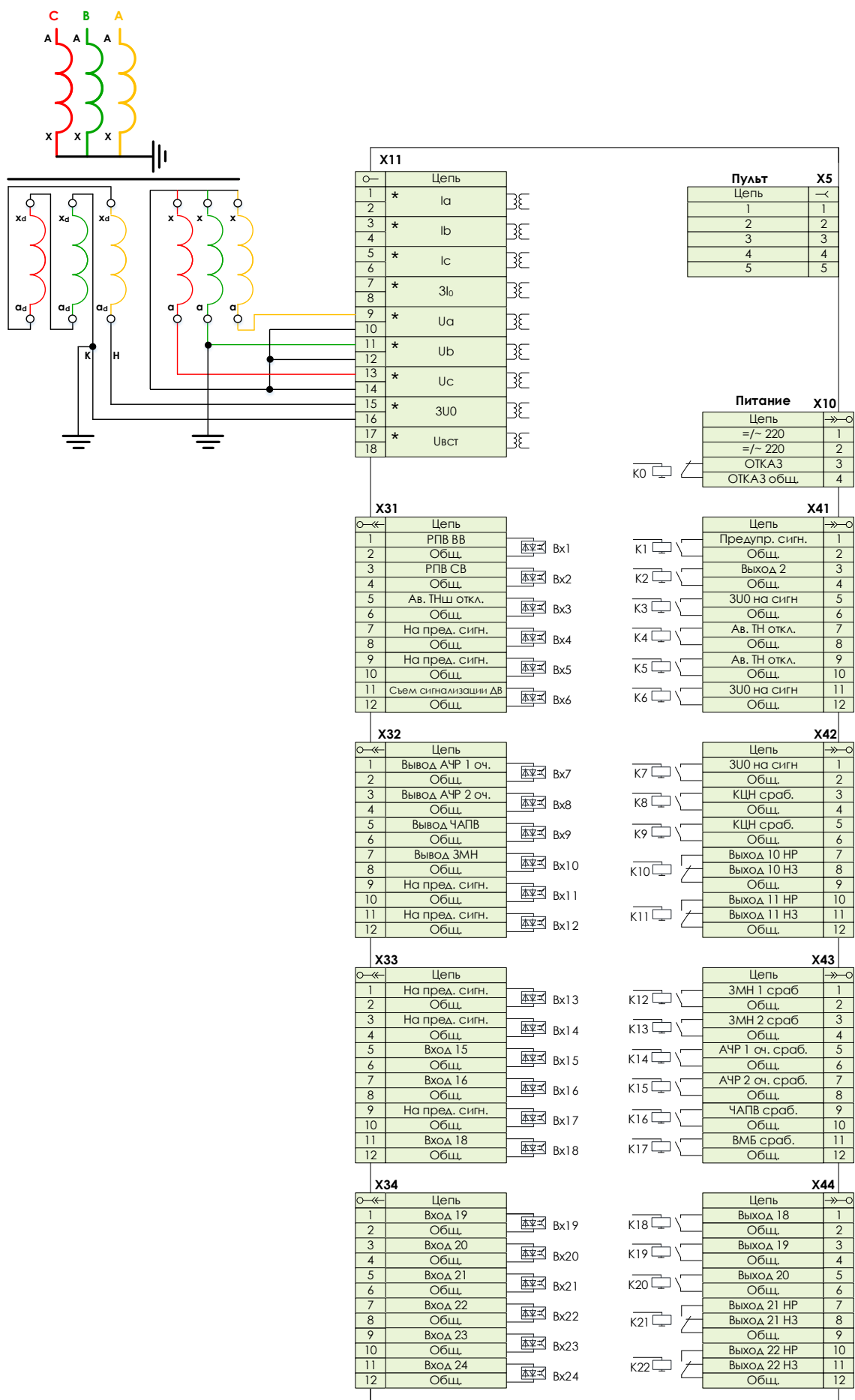
Рисунок 14.7 – Трансформатор напряжения 6-35 кВ
