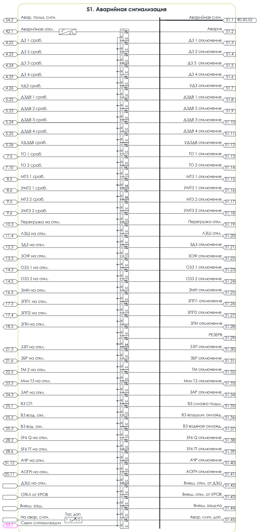
Рисунок 13.4 – Схема №51. Алгоритм аварийной сигнализации
