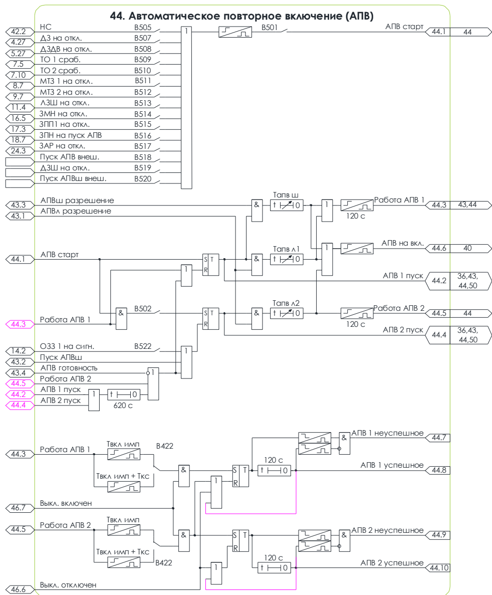
Рисунок 11.6 – Схема №44. Алгоритм АПВ
