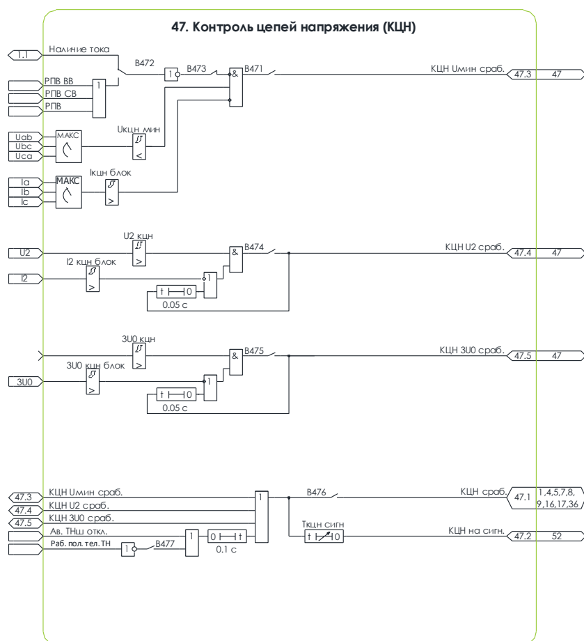
Рисунок 12.2 – Схема №47. Алгоритм КЦН
