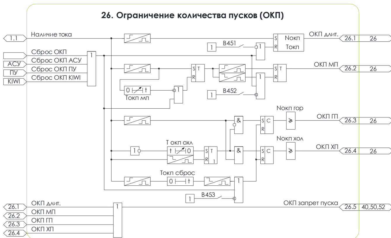
Рисунок 7.7 – Схема №26. Алгоритм ОКП
