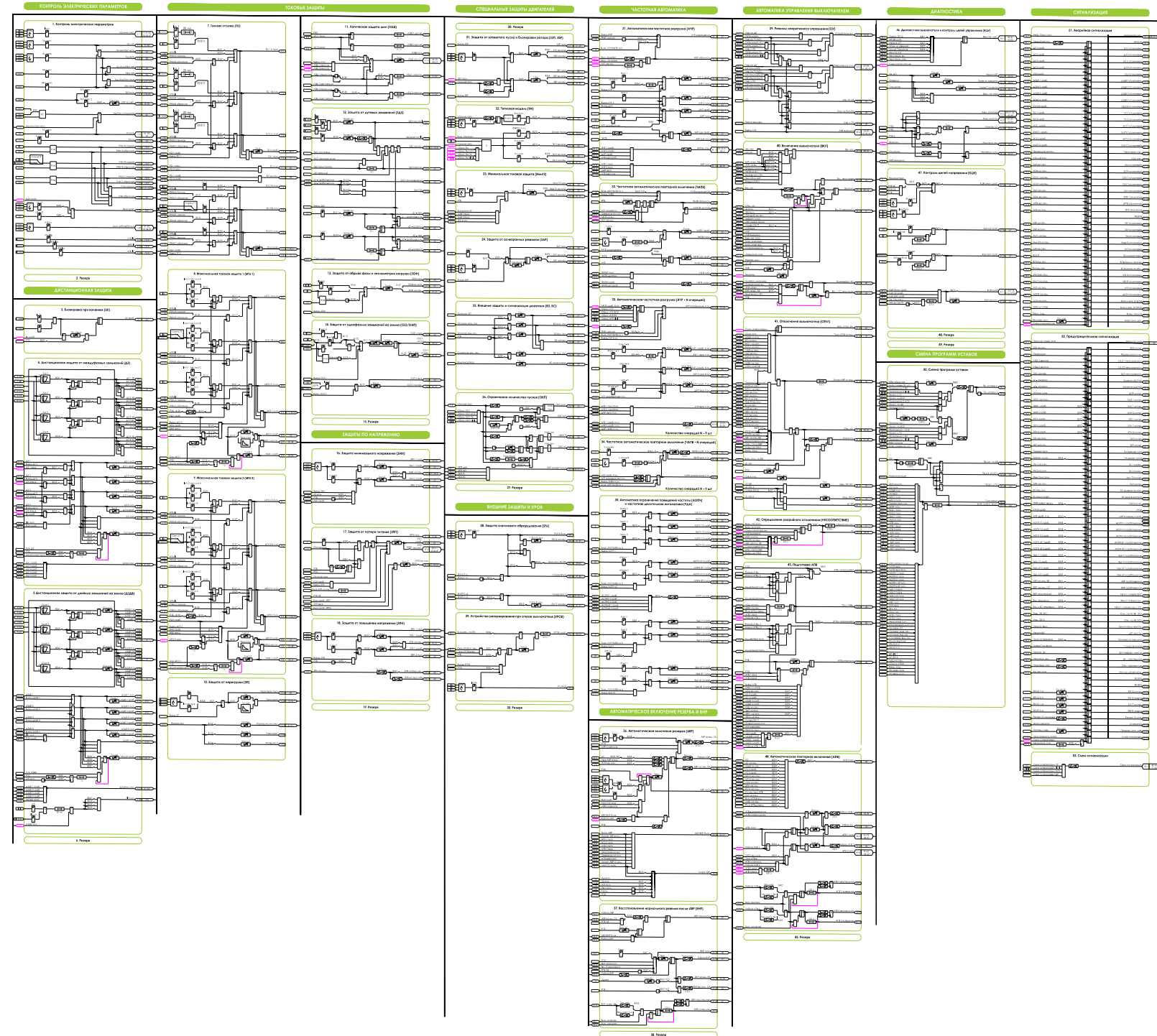
Рисунок Алгоритмы функционирования устройства
