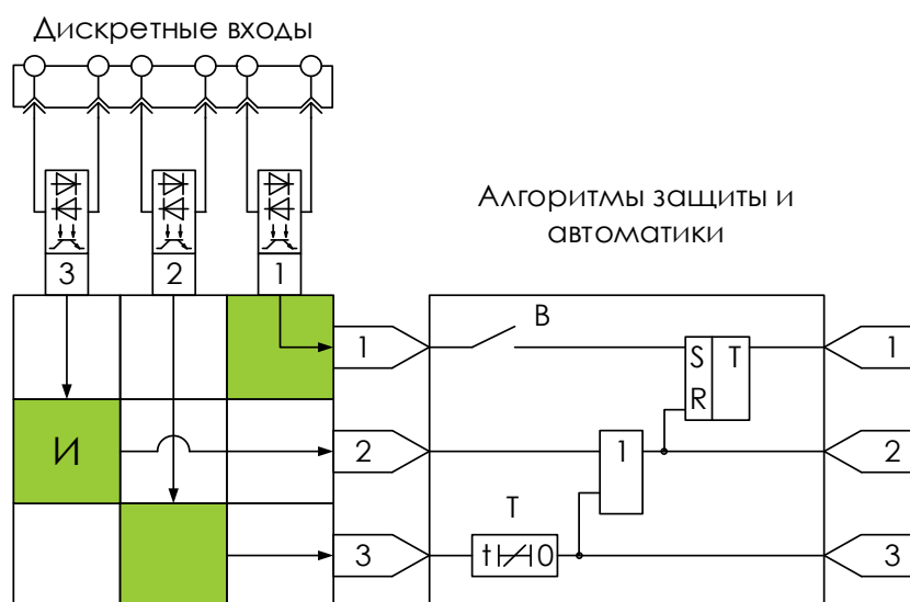
Рисунок 14.10 – Подключение дискретных входов
