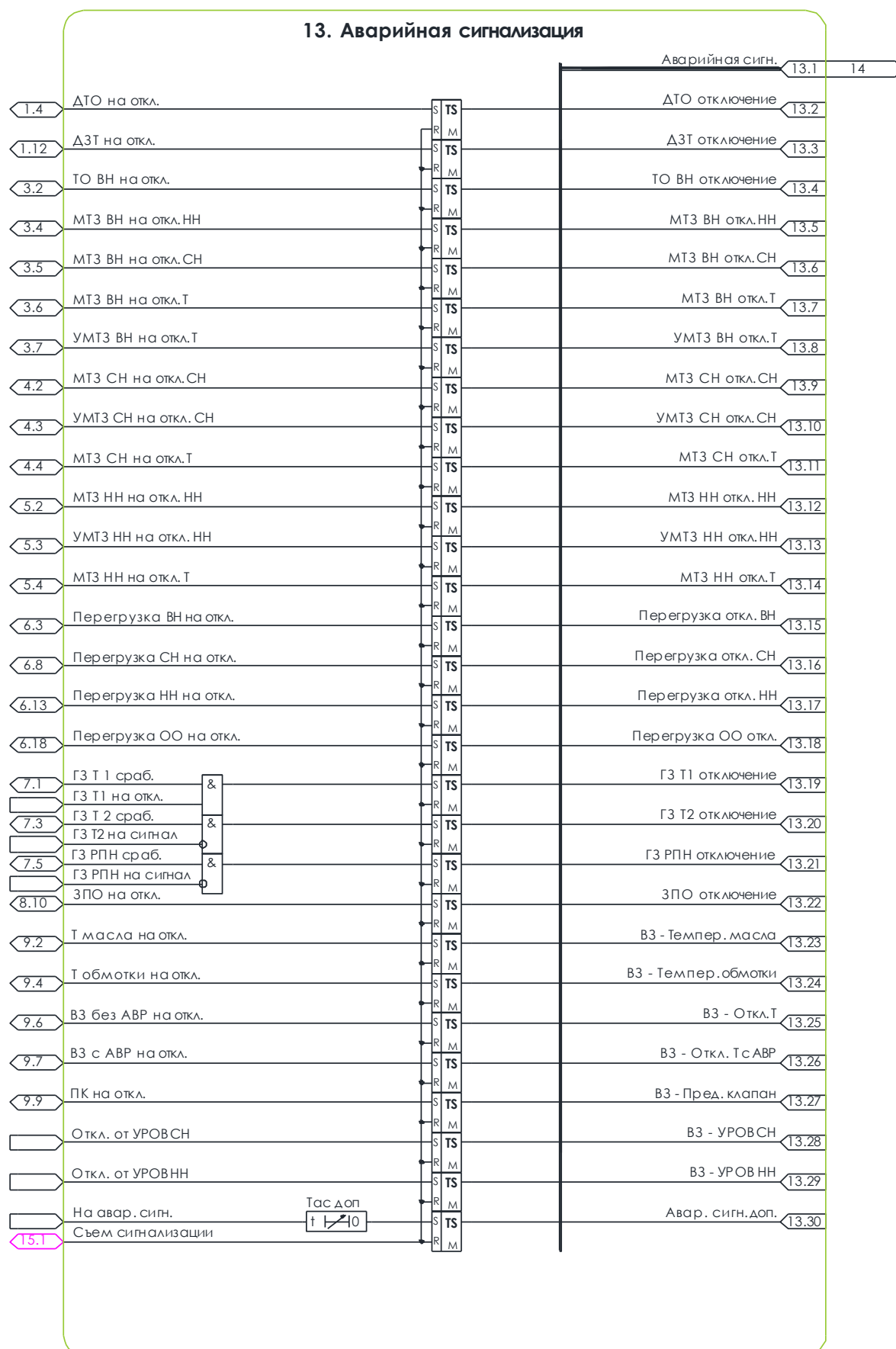
Рисунок 4.3 – Схема №13. Алгоритм аварийной сигнализации
