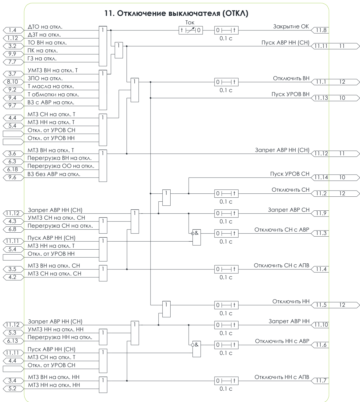
Рисунок 3.15 – Схема №11. Алгоритм отключения выключателя
