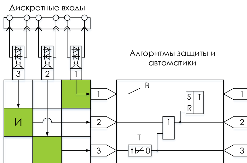
Рисунок 5.7 – Подключение дискретных входов
