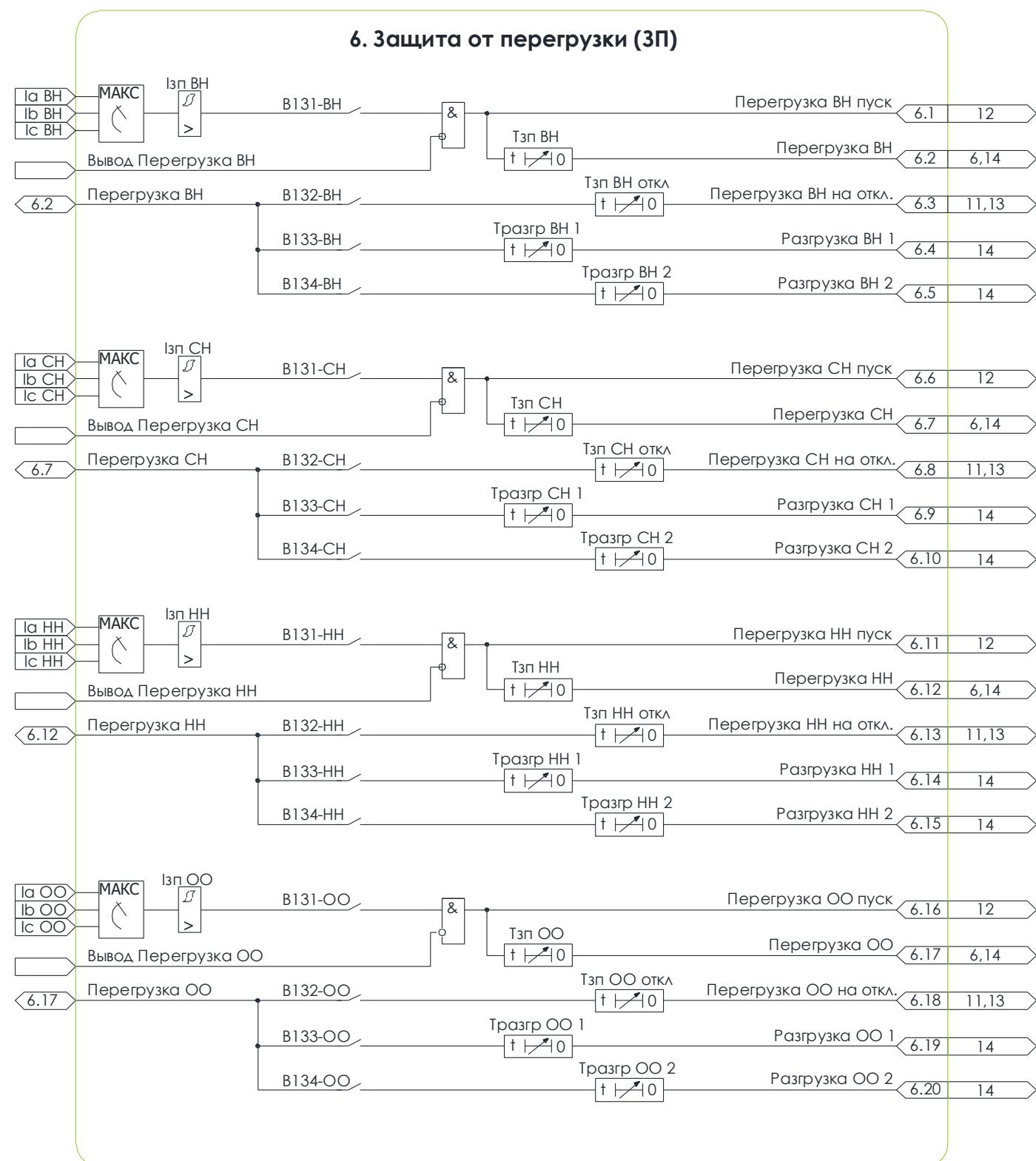
Рисунок 3.9 – Схема №6. Алгоритм ЗП
