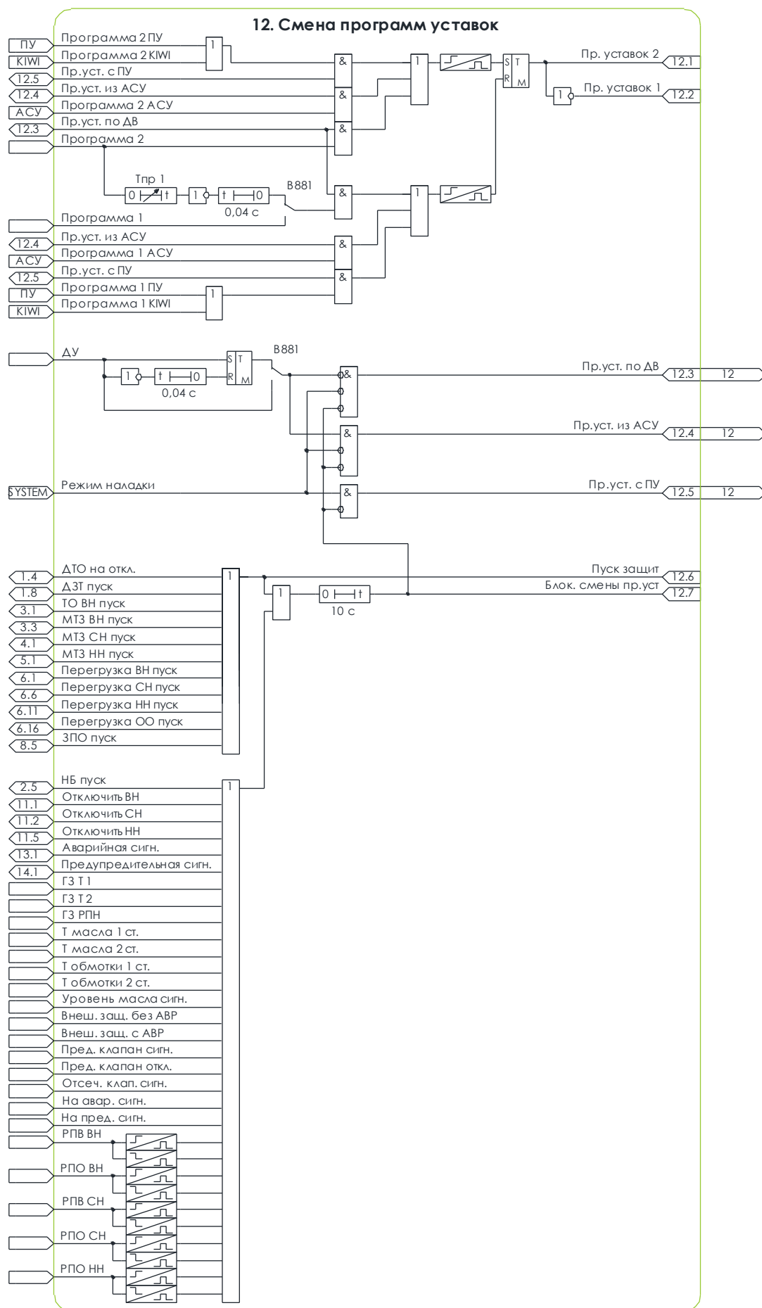
Рисунок 4.1 – Схема №12. Алгоритм выбора программы уставок
