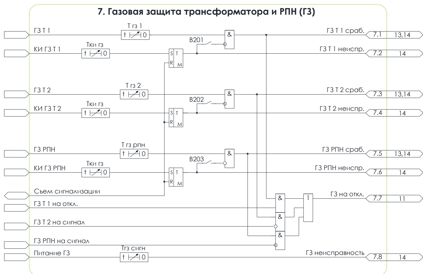
Рисунок 3.10 – Схема №7. Алгоритм ГЗ
