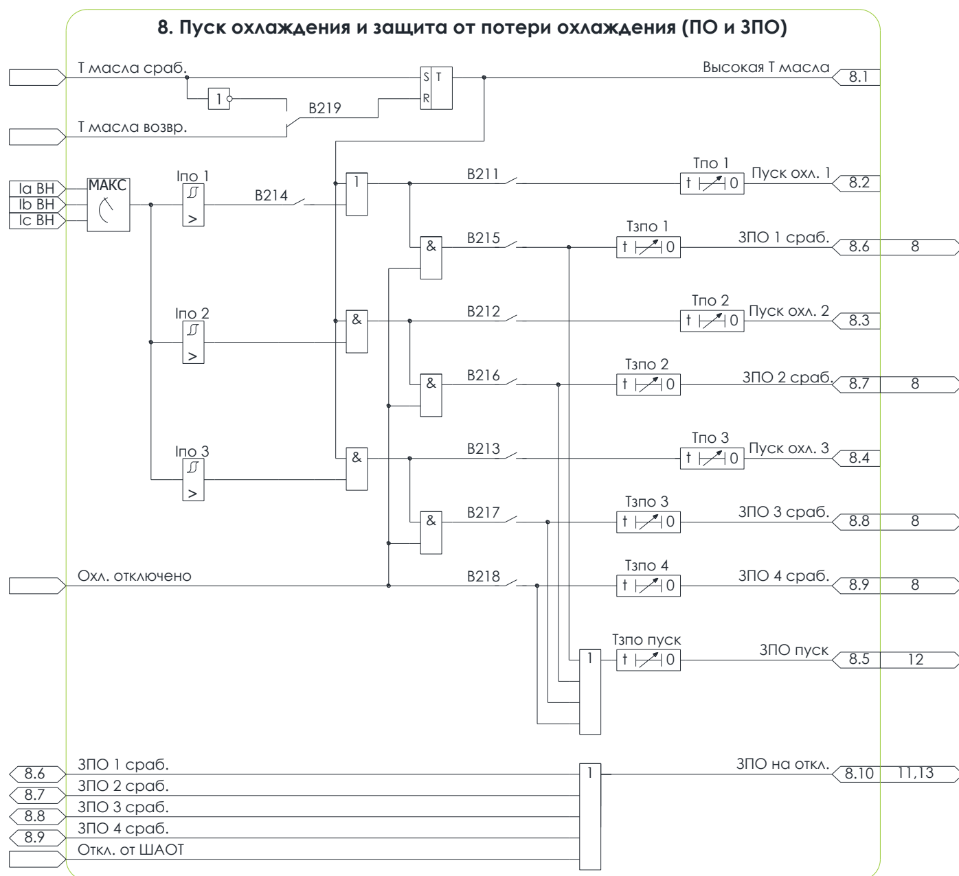
Рисунок 3.12 – Схема №8. Алгоритм ПО и ЗПО
