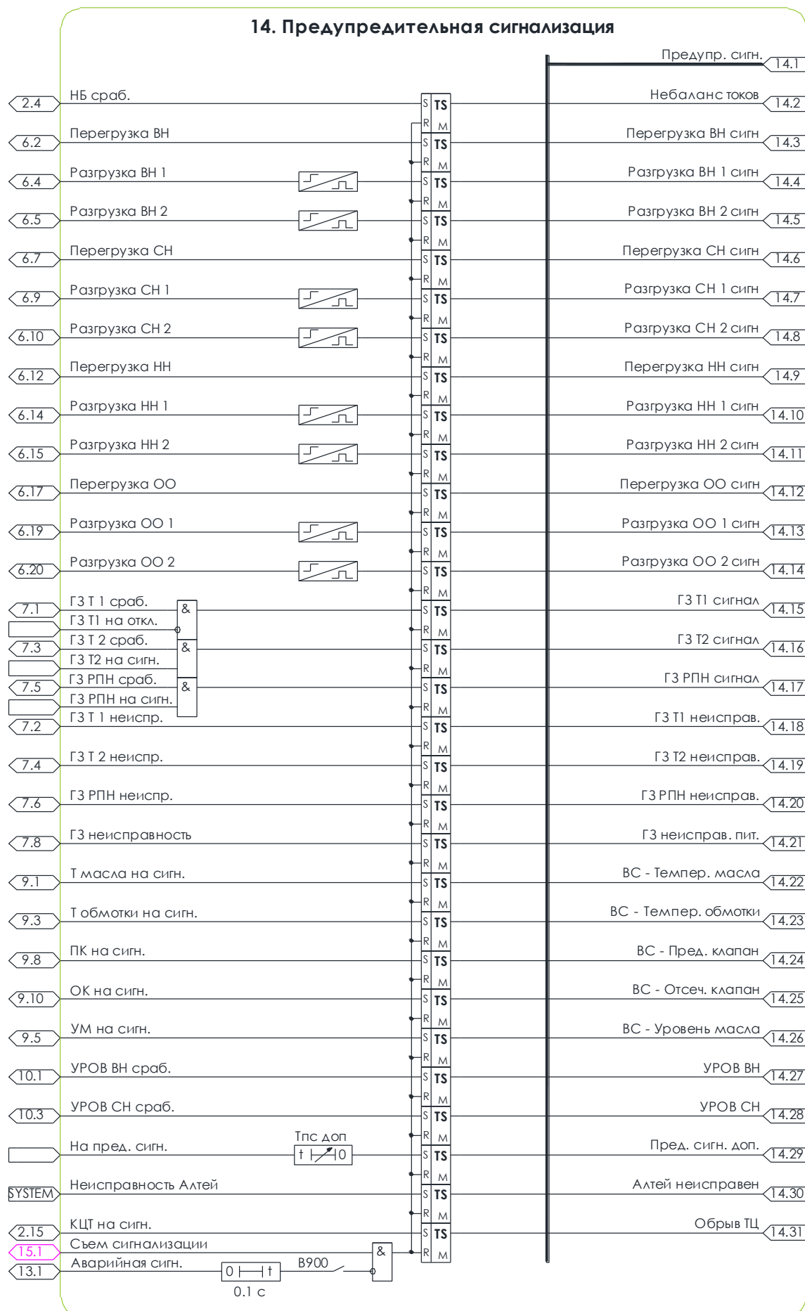
Рисунок 4.4 – Схема №14. Алгоритм предупредительной сигнализации
