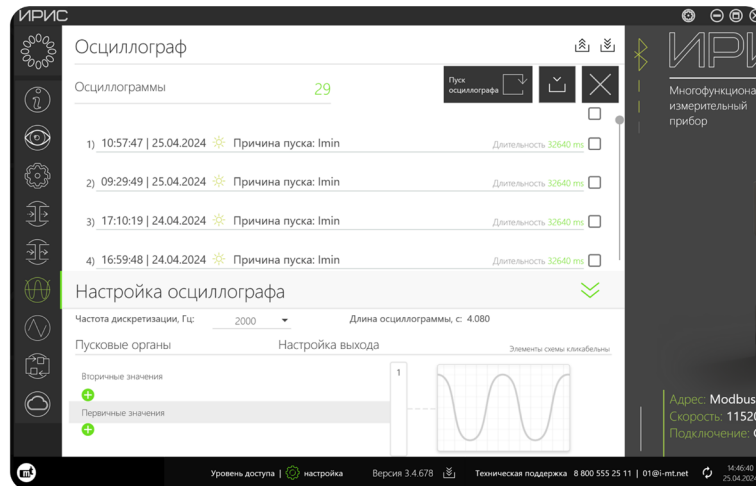
Запись осциллограмм
