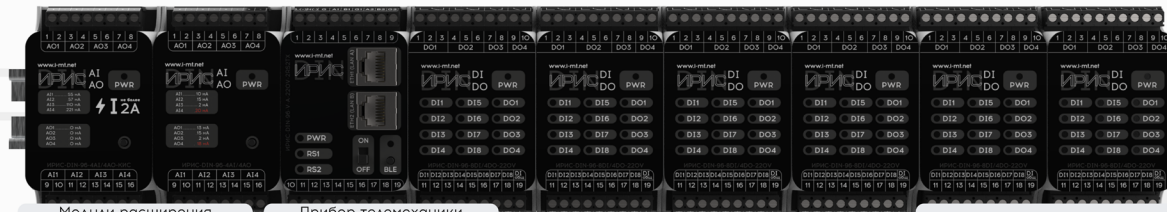
Модули расширения дискретных сигналов 48 входов/24 выхода
