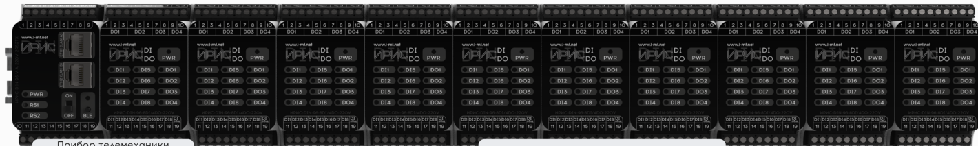
Модули расширения дискретных сигналов 80 входов/40 выходов
