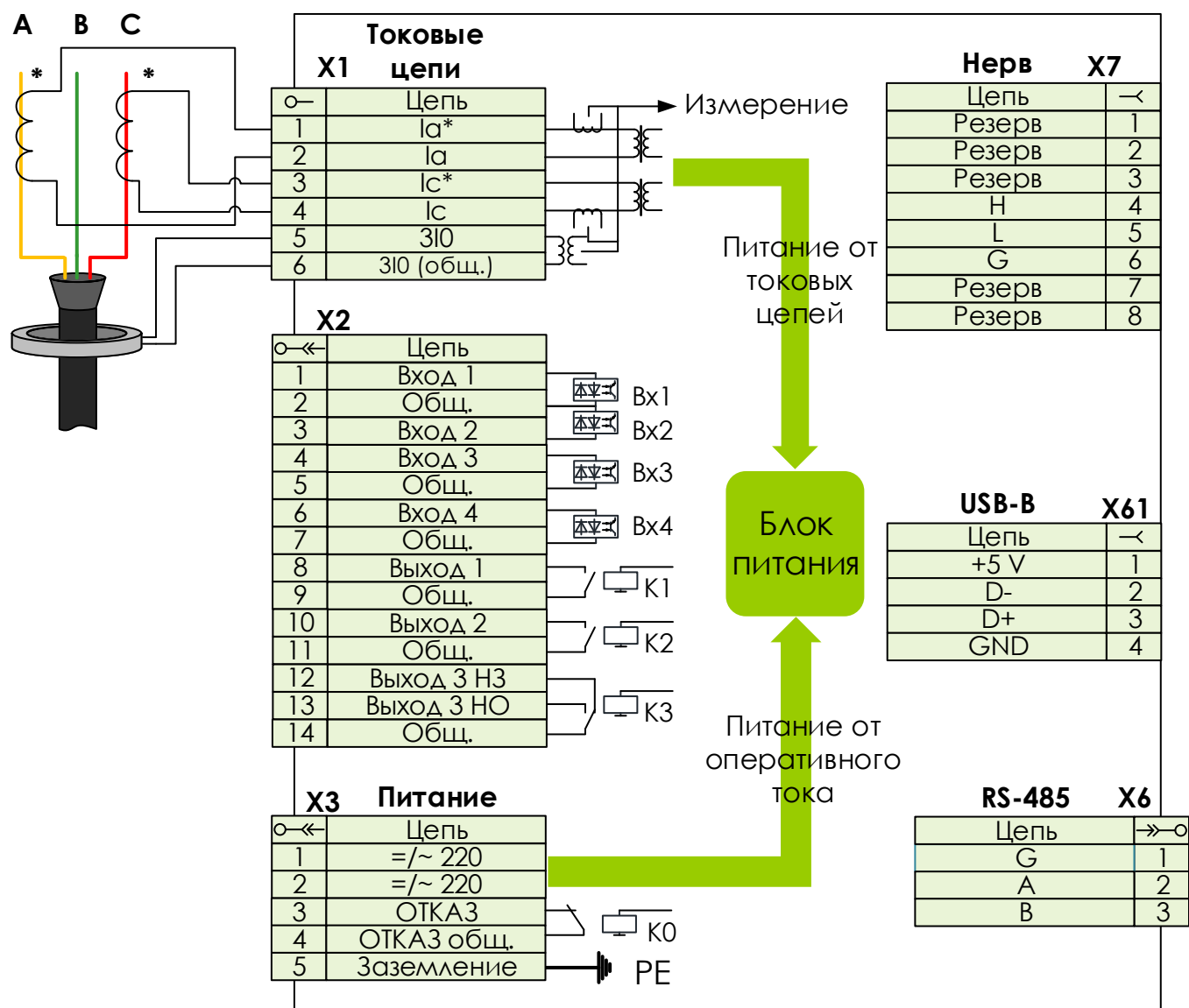
Рисунок П6.2 – Схема электрическая подключения устройств версий 1.XX и 2.XX
