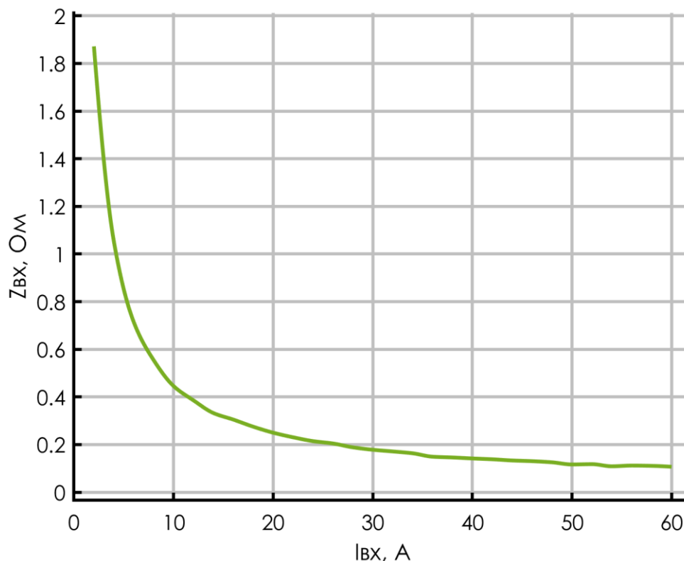
Рисунок 5.1 – Полное сопротивление токового входа блока при отсутствии нагрузки на встроенный источник питания дискретных входов, разомкнутых дискретных выходах, несработанном состоянии модуля дешунтирования
