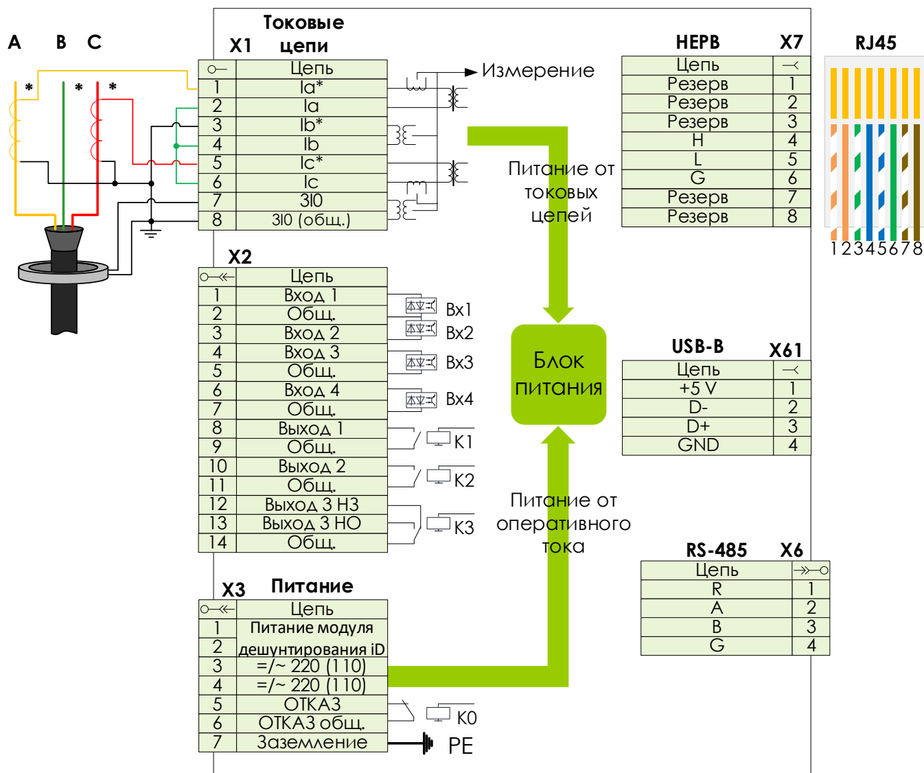
Рисунок 8.4 – Схема электрическая подключения Люттик, Люттик-110 для схемы с двумя ТТ
