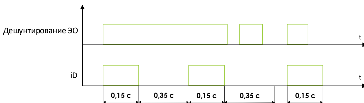
Рисунок П4.1 – Формирование напряжения управления модулем дешунтирования
