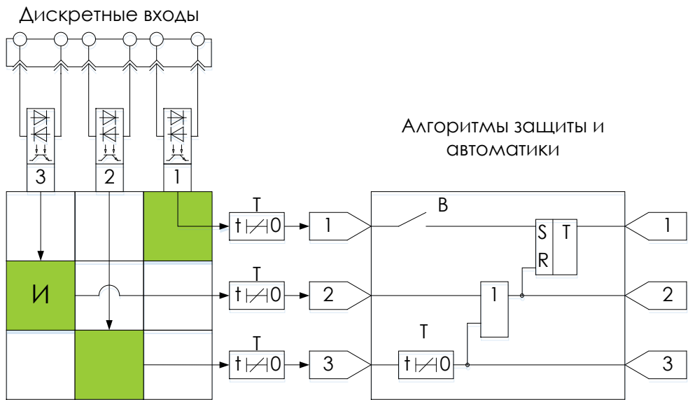
Рисунок 8.7 – Подключение дискретных входов
