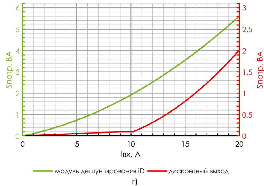
Рисунок 5.2 – Мощность: а,б) потребляемая устройством при разомкнутых дискретных выходах, несрабатанном состоянии модуля дешунтирования; в), г) – потребляемая различной нагрузкой (модулем дешунтирования*, дискретным выходом).
