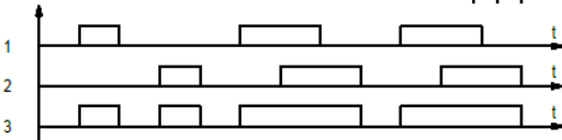
Логическое "ИЛИ"
