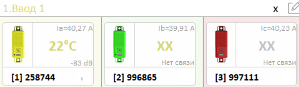
Рисунок 6.20 – KIWI. Настройки Мелиссы. Особенности индикации показаний датчиков
