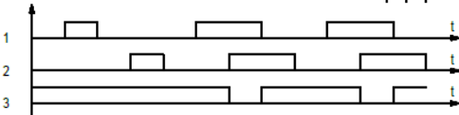
Логическое "И-НЕ"
