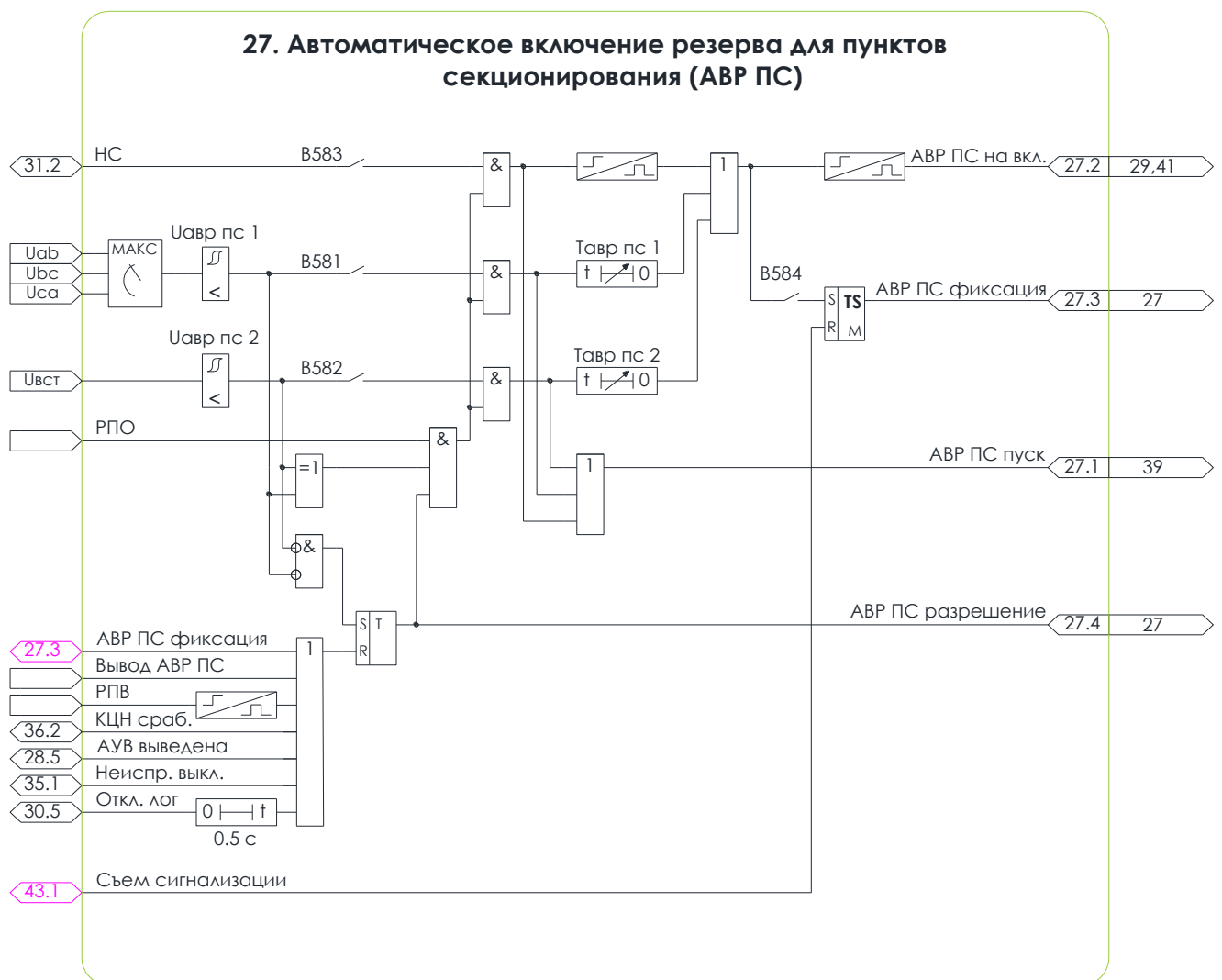
Рисунок 5.25 – Схема №25. Алгоритм АВР ПС
