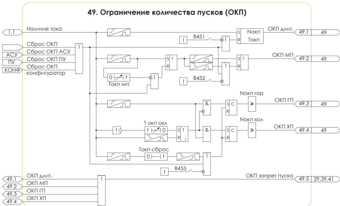
Рисунок 5.39 – Схема №49. Алгоритм ОКП
