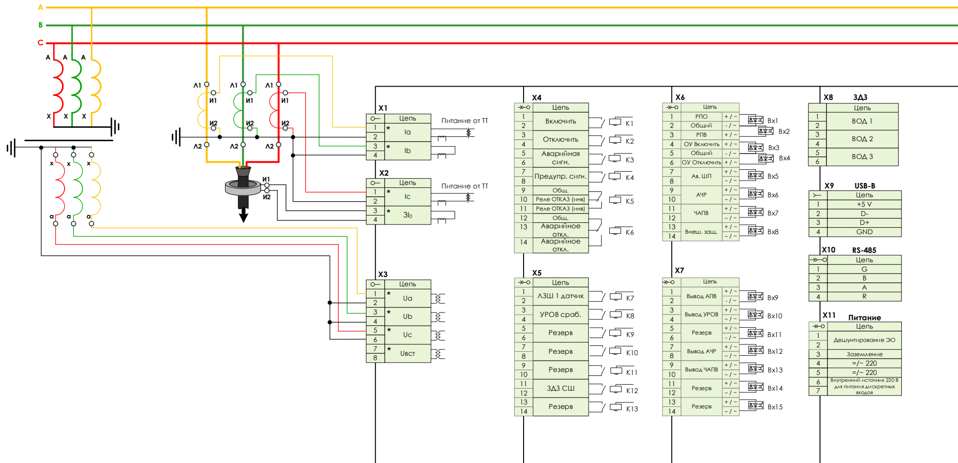
Рисунок Б.6 – Защита на отходящей линии (модификация устройства по дискретным входам/выходам - IO)
