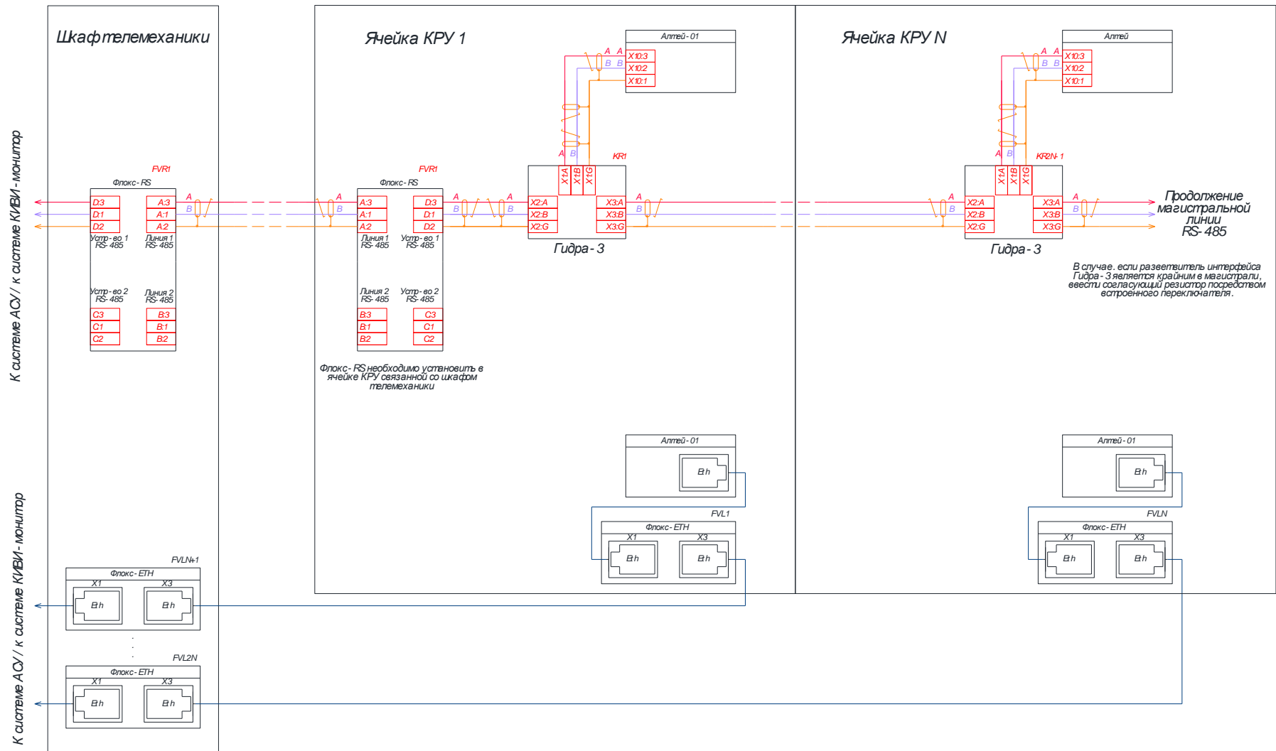
Рисунок 3.1 – Схема организации линий связи интерфейсов RS-485, Ethernet с применением устройств Гидра-3, Флокс-RS, Флокс-ETH
