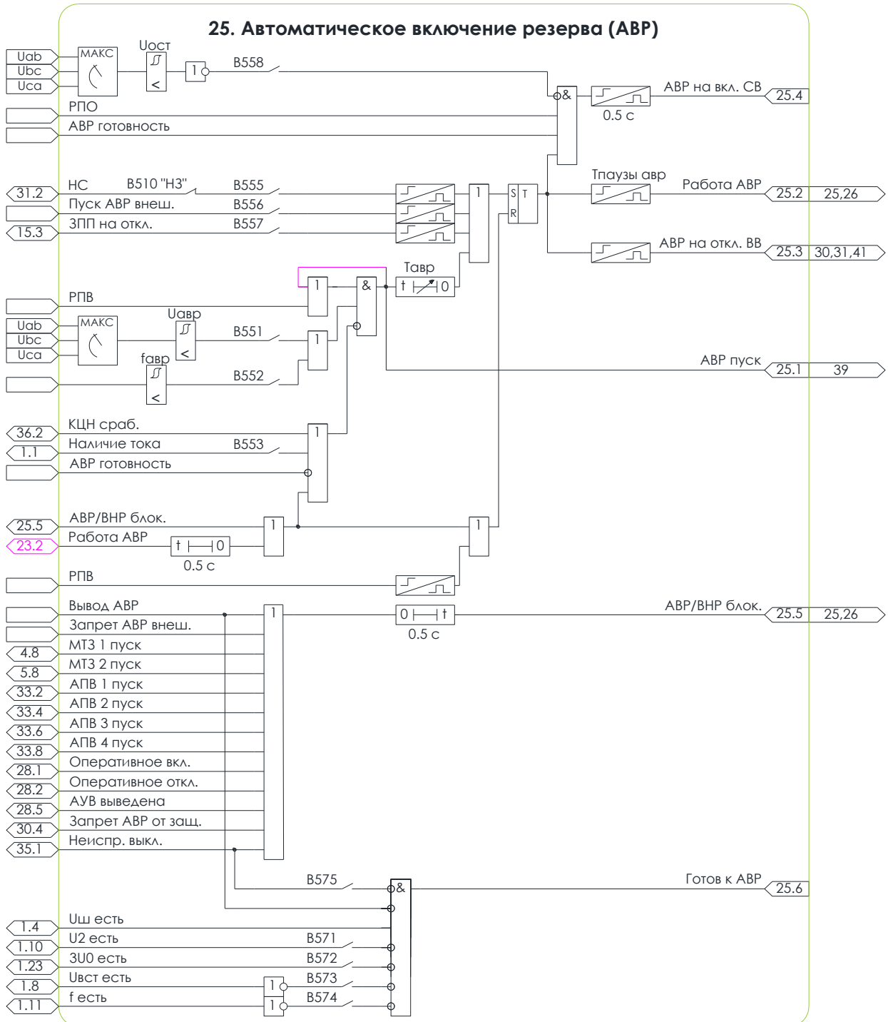
Рисунок 5.23 – Схема №25. Алгоритм АВР
