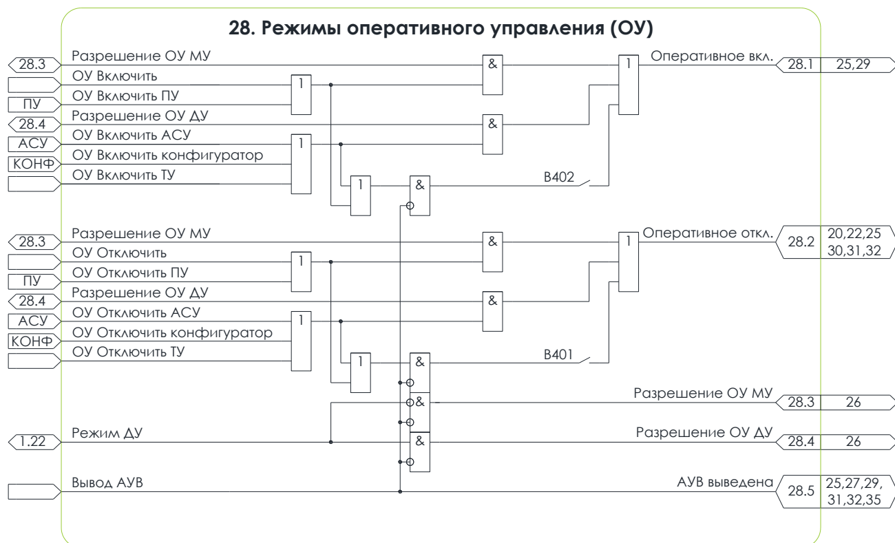
Рисунок 5.26 – Схема №28. Алгоритм ОУ
